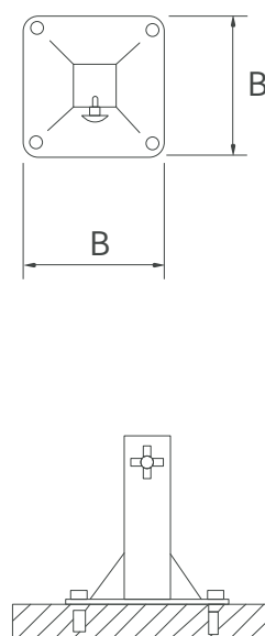
Detalle base pletina
