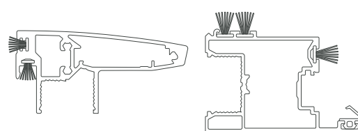
Detalle perfil marco abatible
