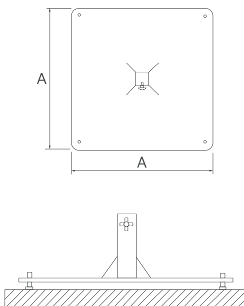
Detalle base de lastre
