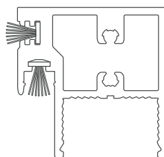
Detalle perfil marco
